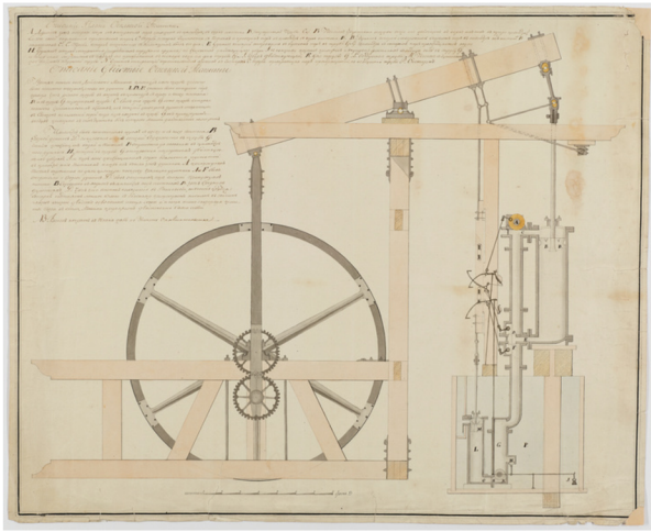
Höyrykoneen piirustus. (Museovirasto)
